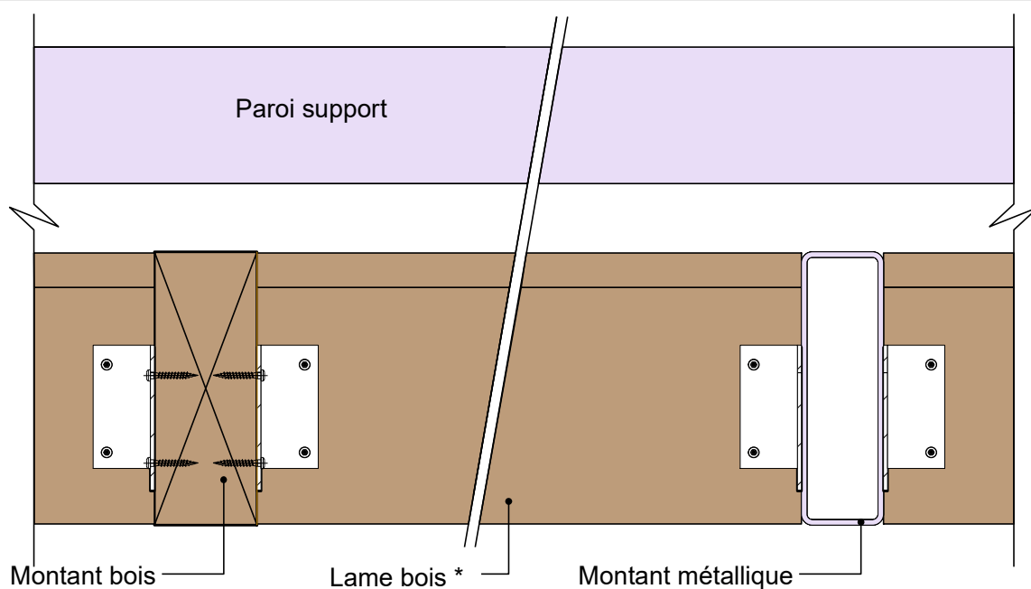
Coupe horizontale
