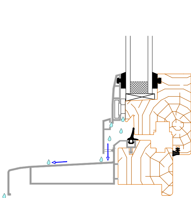
Systèmes de menuiseries mixtes bois-aluminium à liaison mixte étanche
