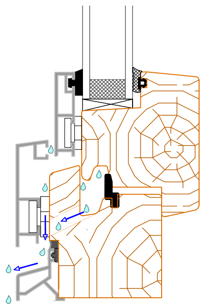
Systèmes de menuiseries mixtes bois-aluminium à liaison mixte étanche
