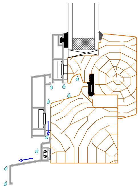
Traverse basse avec bavette aluminium
