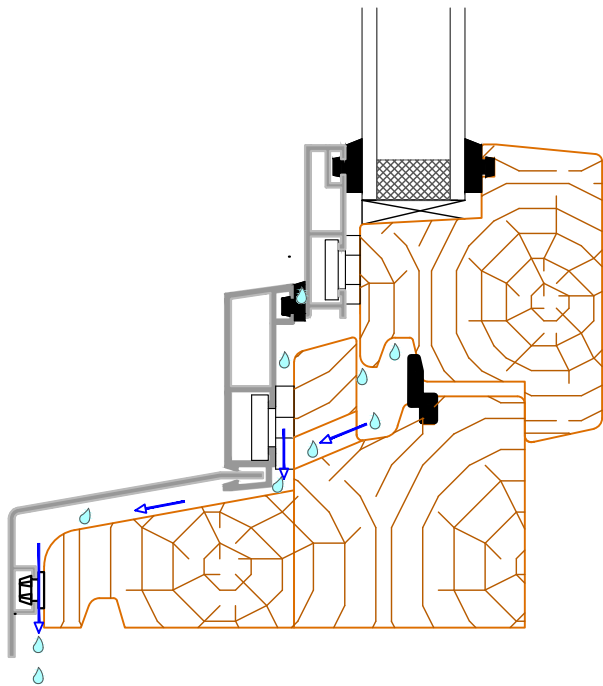
Nez d'appui rapporté + capotage aluminium
