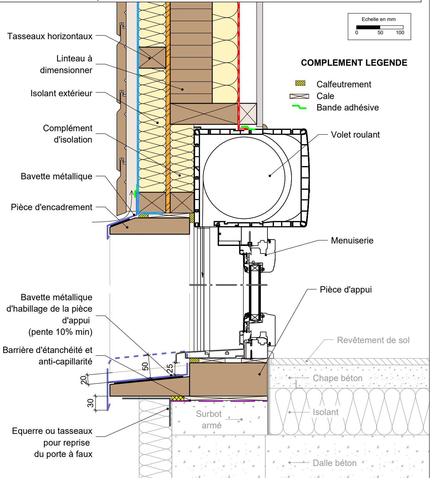
MUR EXTERIEUR TYPE 6: Isolant en âme et en doublage extérieur Détail sur porte-fenêtre bois-alu et volet roulant
