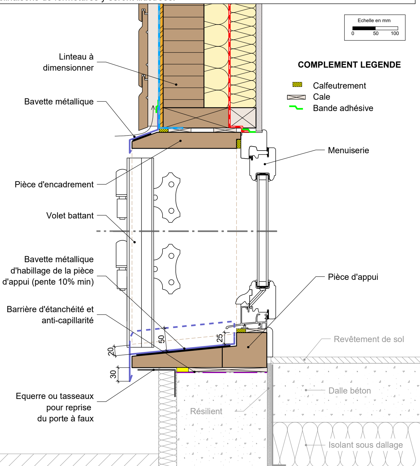
MUR EXTERIEUR TYPE 4: Isolant en âme et doublage intérieur Détail sur porte-fenêtre bois et volet bois
