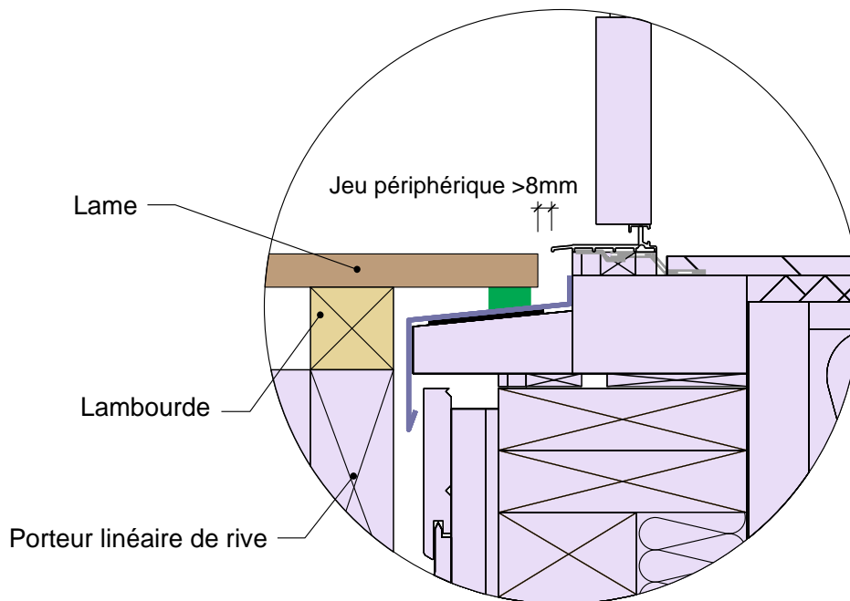
Coupe longitudinale - accès menuiserie PMR (Exemple sur structure bois)
