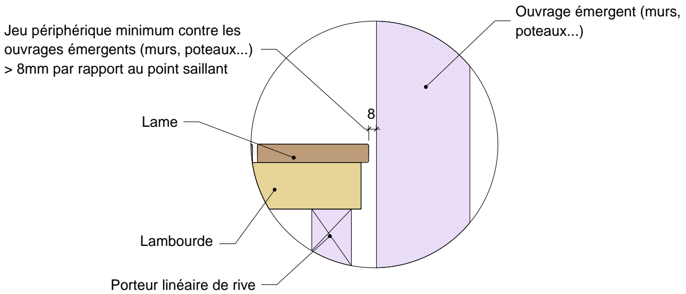
Coupe transversale - partie courante
