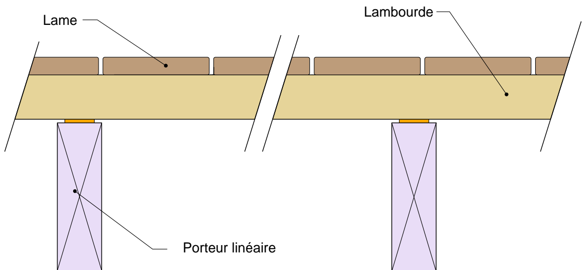
Coupe transversale
