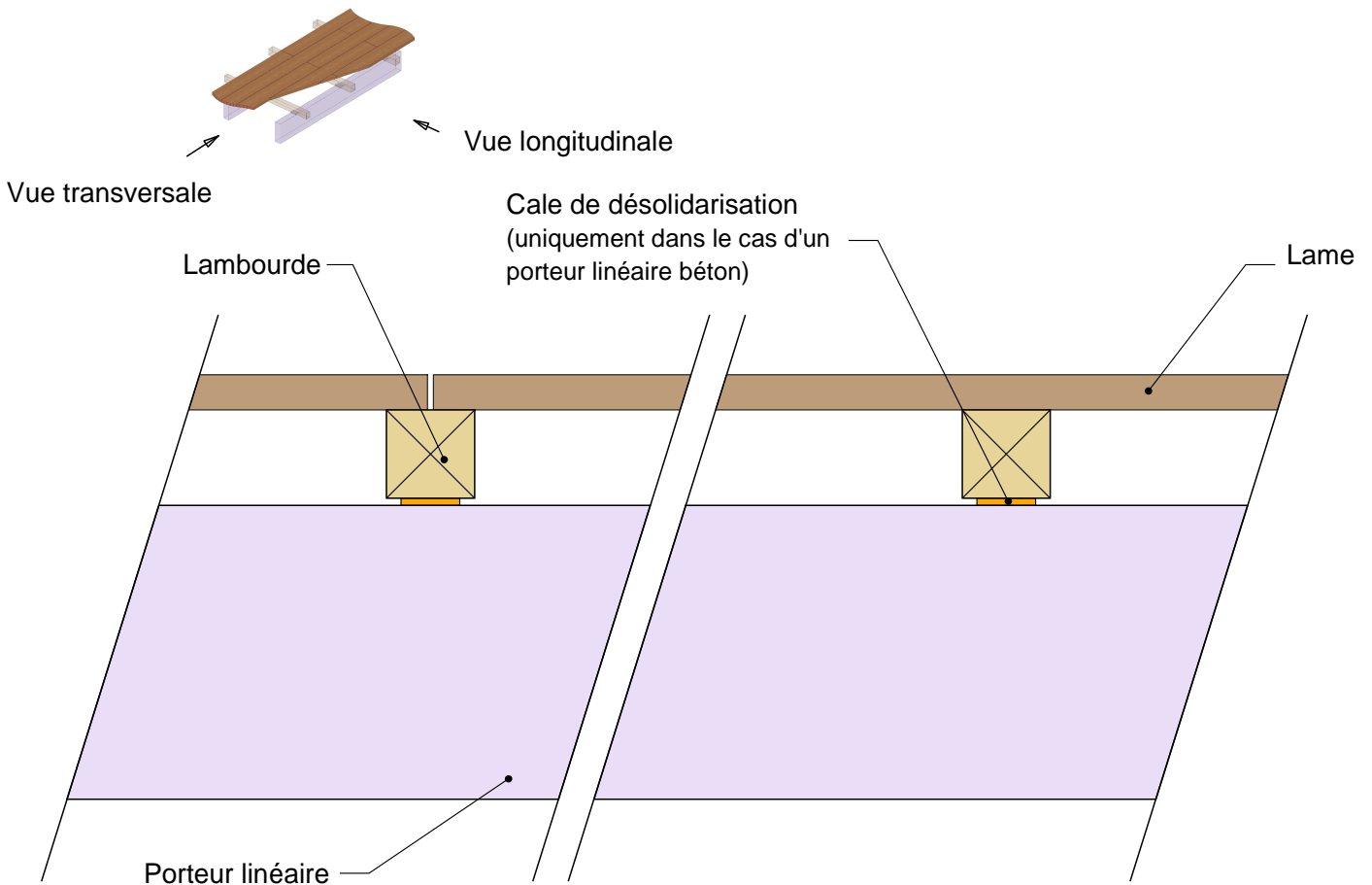
Coupe longitudinale
