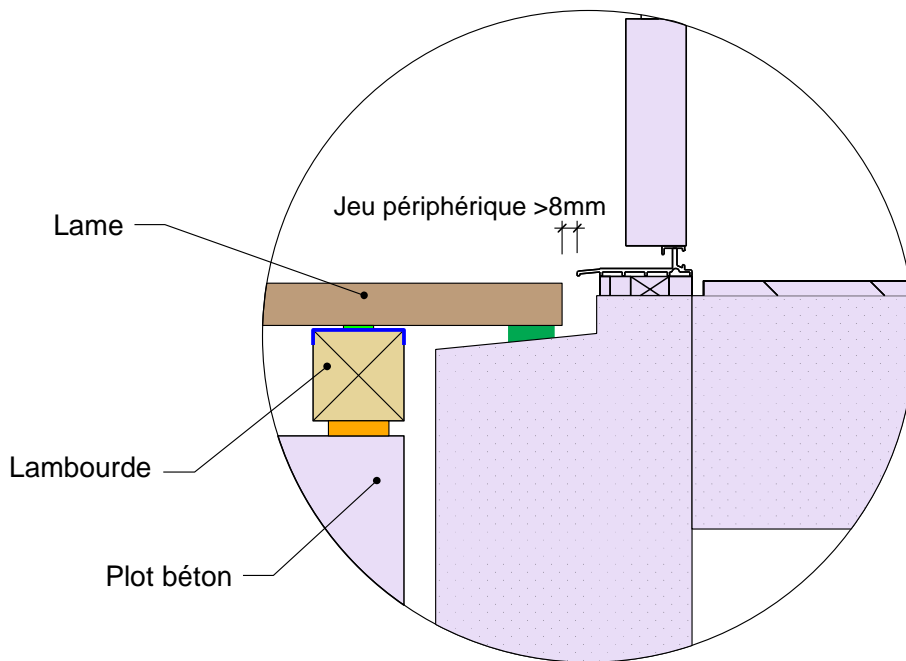
Coupe longitudinale - accès menuiserie PMR
