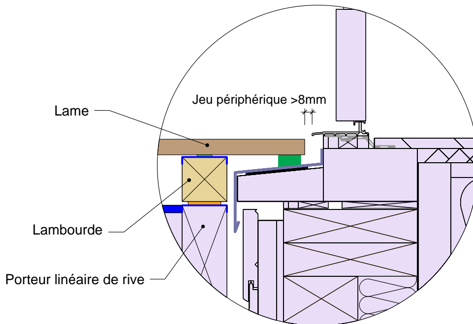
Coupe longitudinale - accès menuiserie PMR (Exemple sur structure bois)
