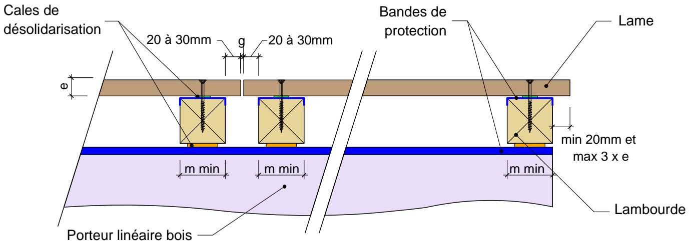
Coupe longitudinale
