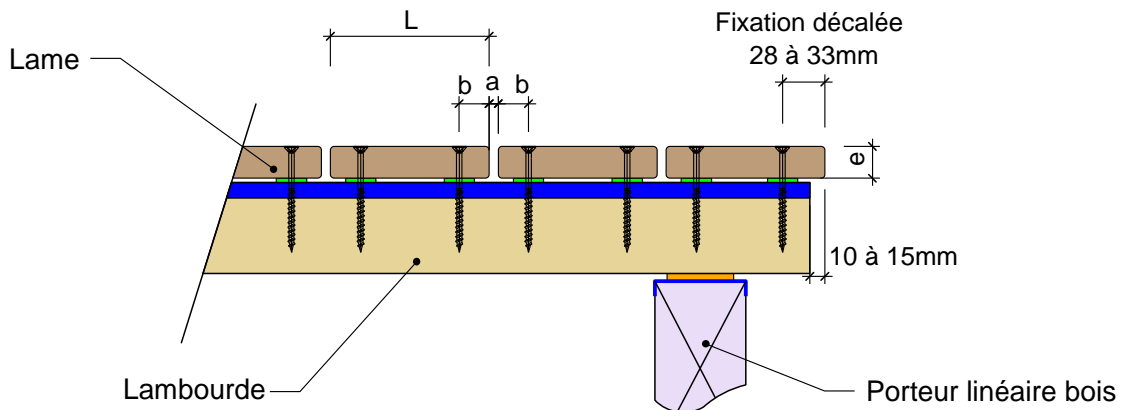
Coupe transversale
