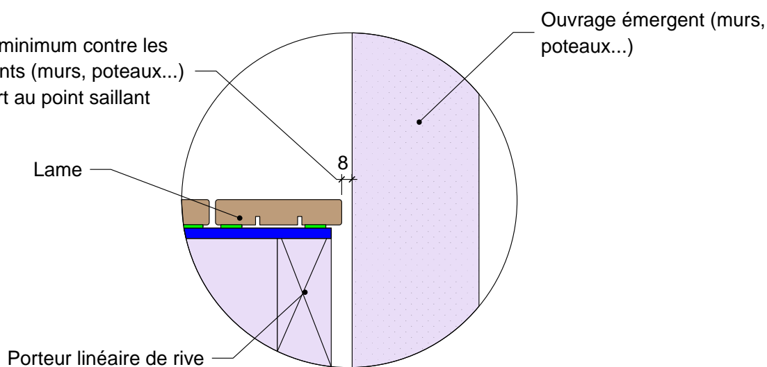
Coupe transversale - partie courante
