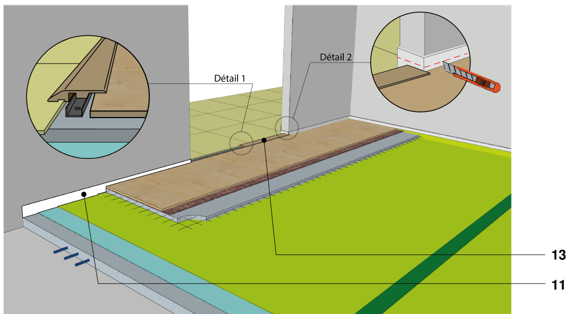
Coupe sur Détail 1
