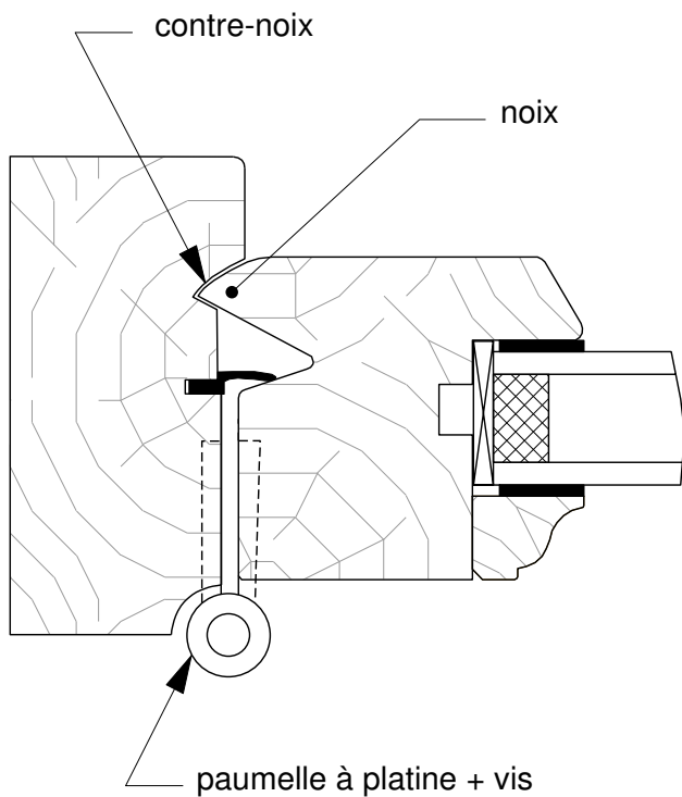
Liaison noix - contre-noix
