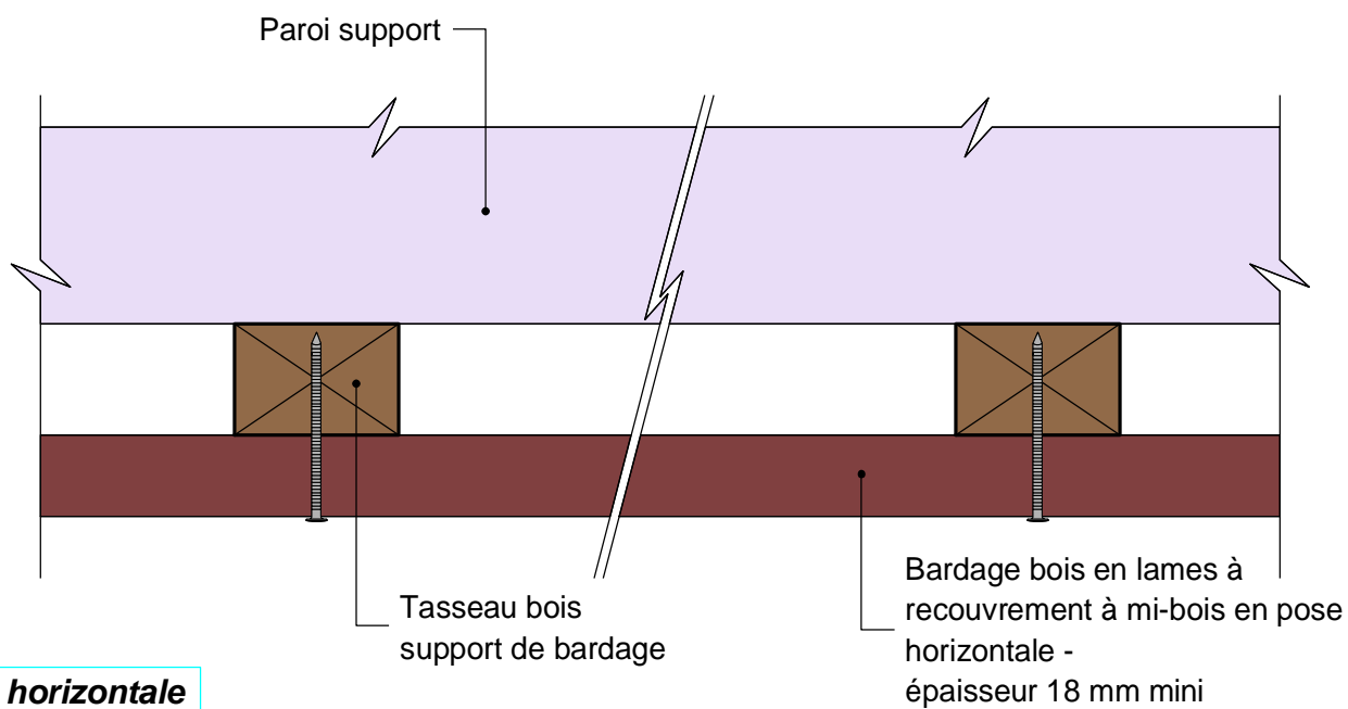
Coupe verticale
