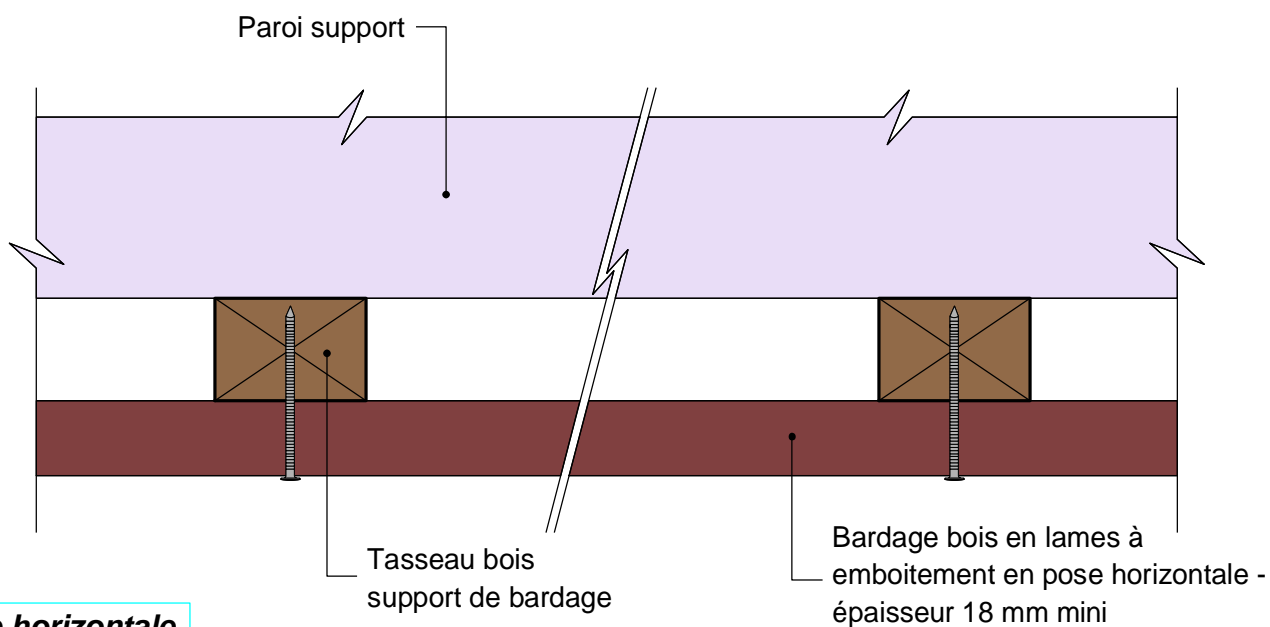
Coupe horizontale
