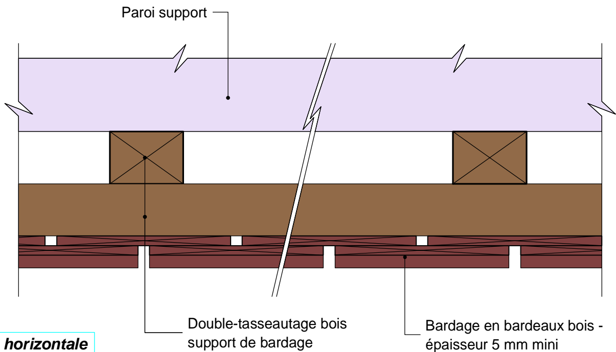
Coupe verticale
