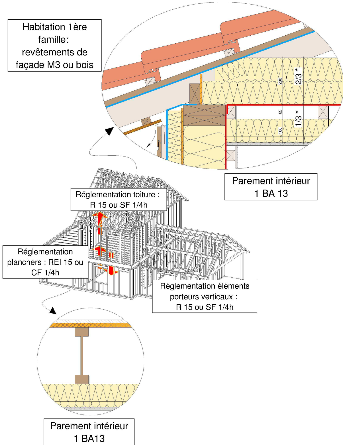
Figure 1: Schéma illustrant la réglementation incendie et des types de parois permettant de répondre à celle-ci pour une maison individuelle type.
