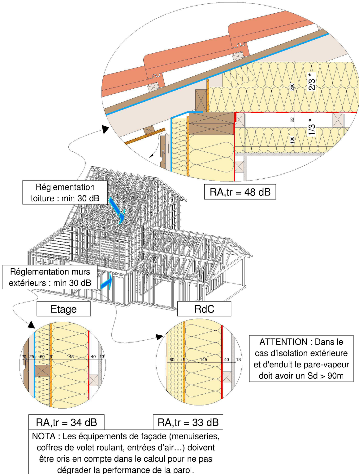
Figure 2: Schéma illustrant la réglementation acoustique et des types de parois pouvant répondre à celle-ci pour une maison individuelle type.
