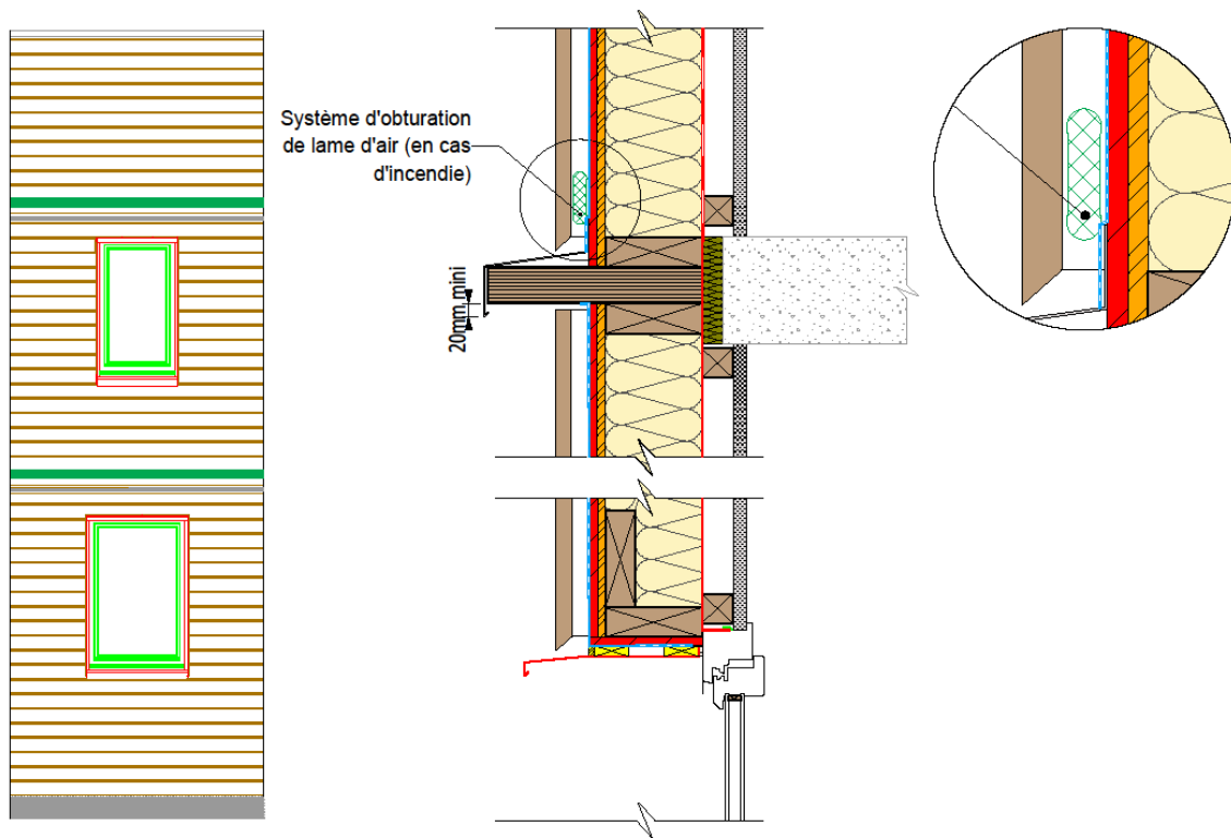
Figure 8 : Position des dispositifs d'obturation de la lame d'air si la durée de résistance au feu de la structure est inférieure ou égale à 60 minutes avec un bardage ventilé dont la performance en réaction au feu du parement est soit de classe D-s2, d0 ou soit de classe C-s2, d0.
