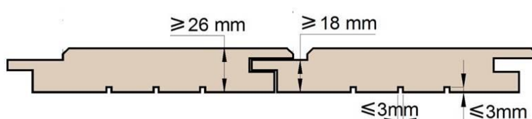
Figure 7: Epaisseurs des profils de bardage – Prescriptions.
