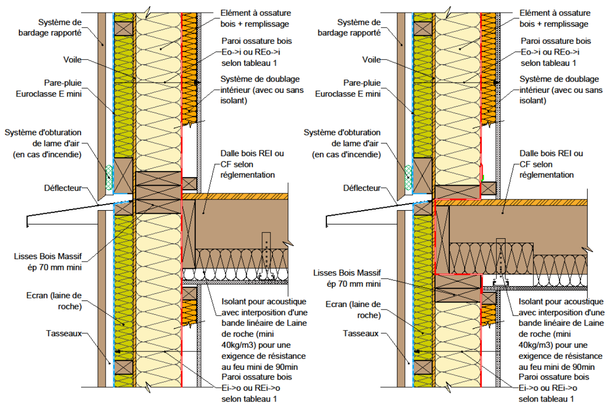
Figure 19 : Façade/mur ossature bois & plancher en ossature bois.
