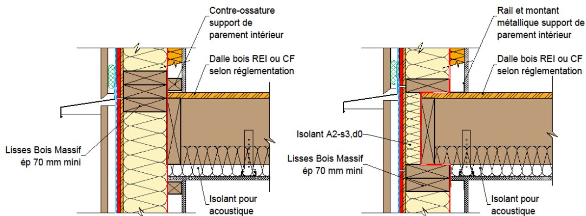
Figure 3: Traitement de l'étanchéité au nez d'un plancher bois avec doublage intérieur assurant l'intégralité de l'exigence EI_{i>0} requise et au moins égale à la performance du plafond (si la durée de résistance au feu de la structure est inférieure ou égale à 60 minutes).
