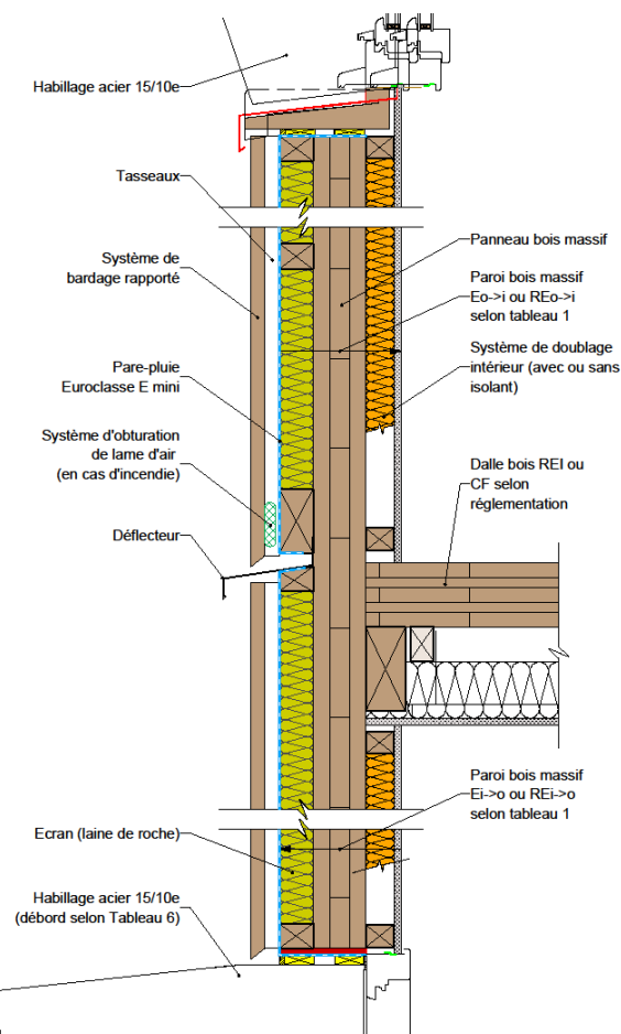
Figure 26 : Façade/mur en panneaux bois massifs & plancher en panneaux bois massifs.
