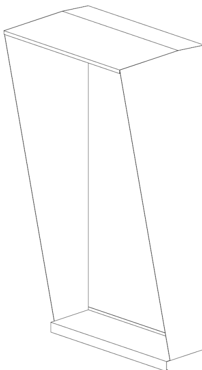
Figure 12 : Habillage en acier des embrasures
