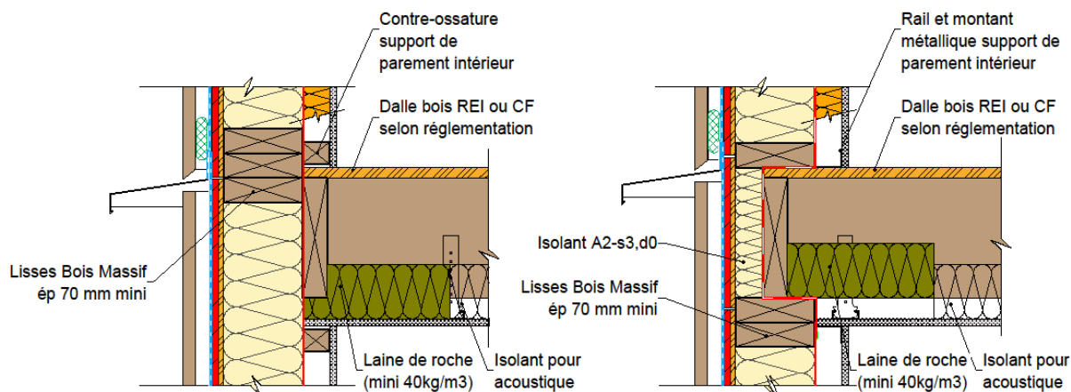
Figure 4: Traitement de l'étanchéité au nez d'un plancher bois avec doublage intérieur assurant l'intégralité de l'exigence EI_{i>0} requise et au moins égale à la performance du plafond (si la durée de résistance au feu de la structure est supérieure ou égale à 90 minutes).
