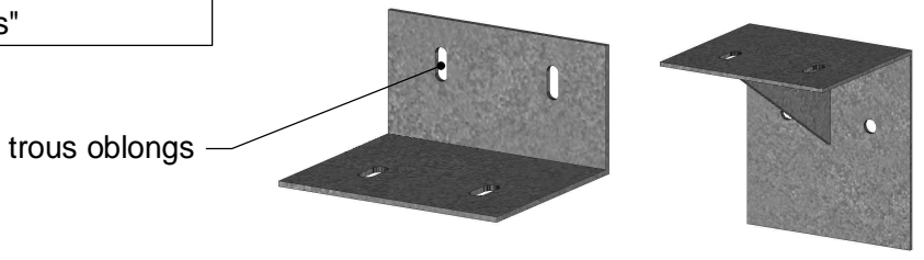
Vue 3D équerres (principe)
