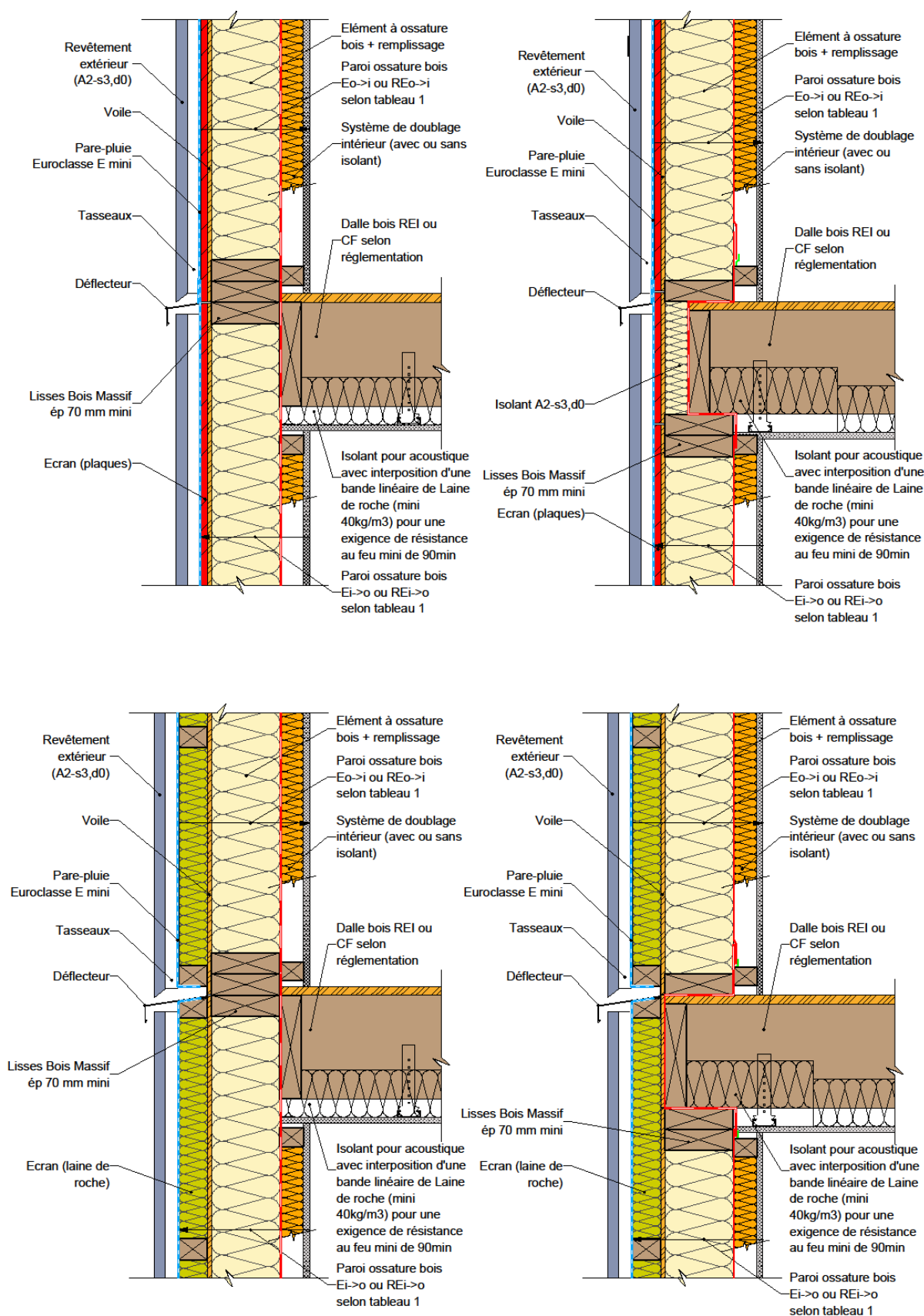
Figure 32 : Façade/mur en ossature bois & plancher en ossature bois.
