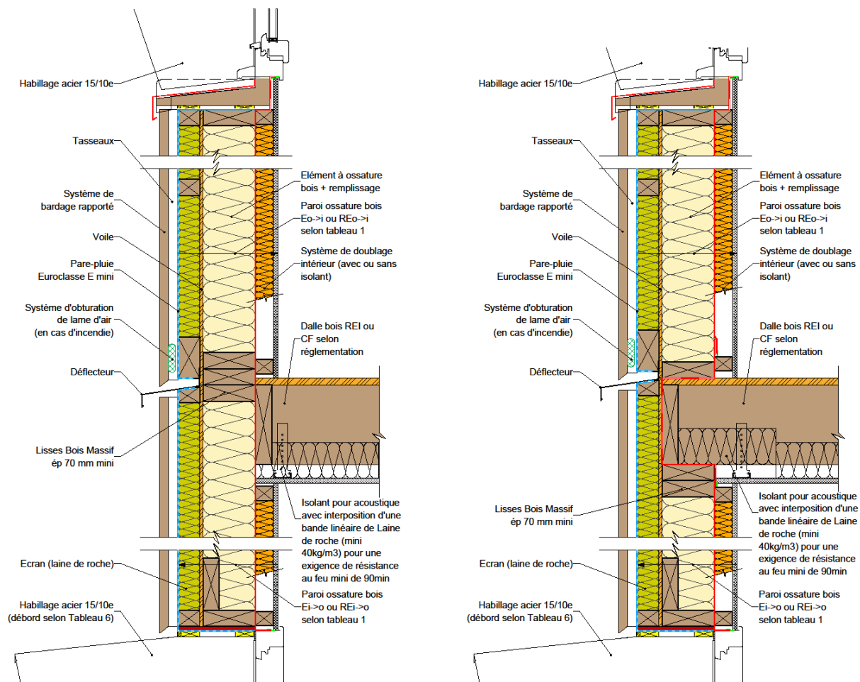
Figure 28 : Façade/mur en ossature bois & plancher en ossature bois.
