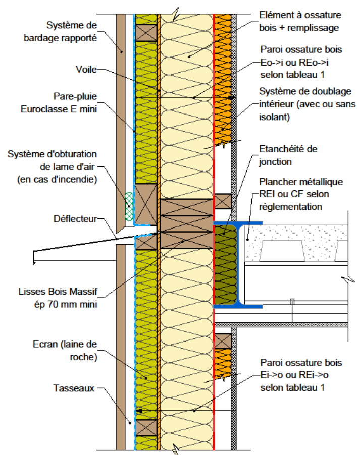
Figure 26 : Façade/mur ossature bois & plancher métallique.
