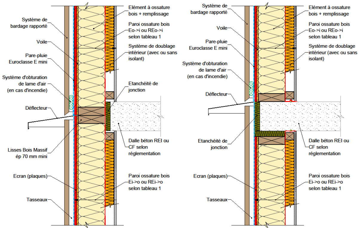
Figure 15 : Façade en ossature bois sur plancher béton.
