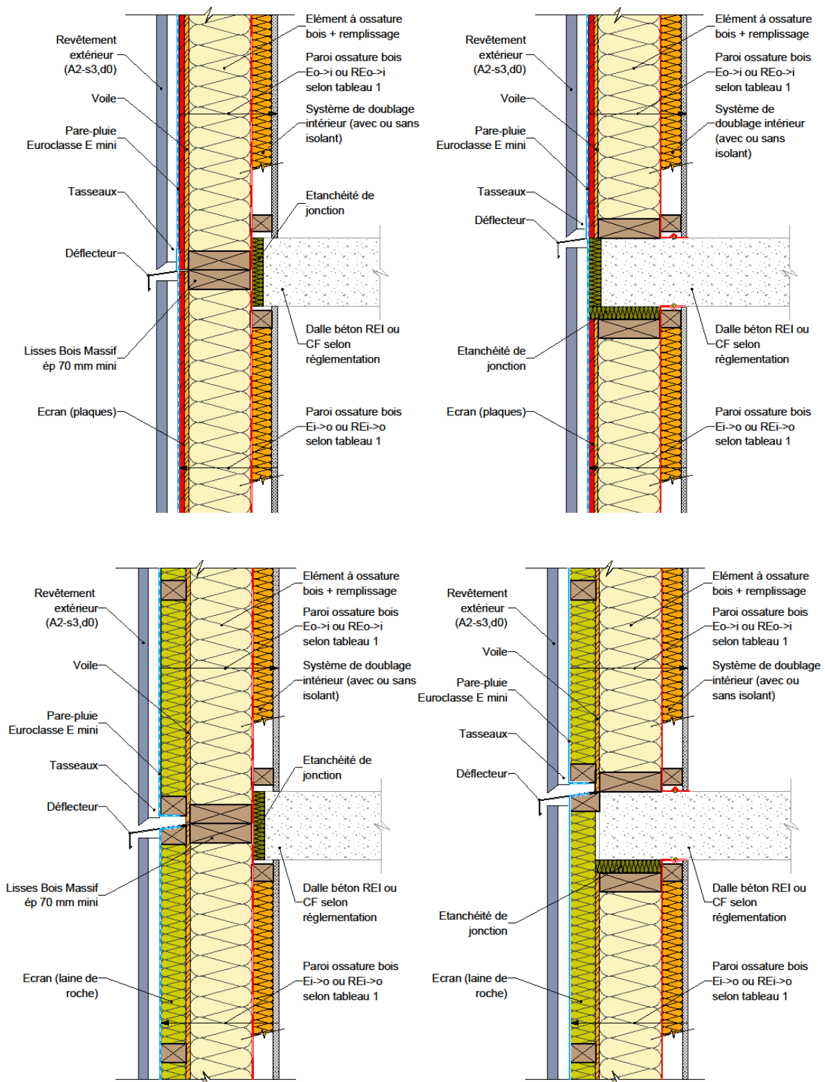
Figure 31 : Façade/mur en ossature bois & plancher en béton.
