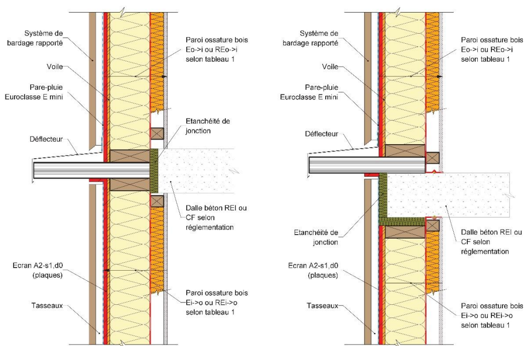
Figure 21 : Exemple de paroi avec déflecteurs renforcés d'une Façade ossature bois sur plancher en béton.
