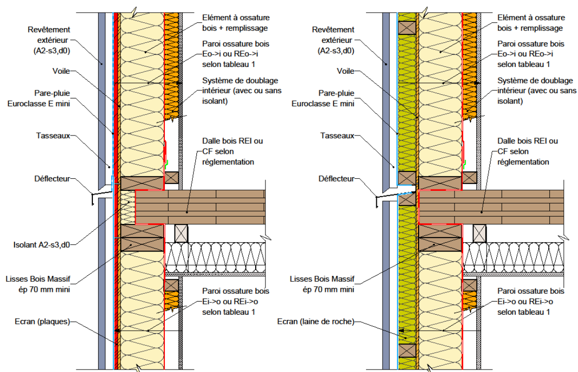
Figure 34 : Façade/mur en ossature bois & plancher en panneaux bois massif.
