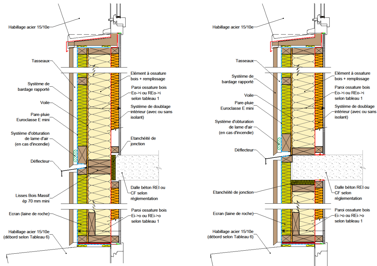
Figure 27 : Façade/mur ossature bois & plancher en béton.
