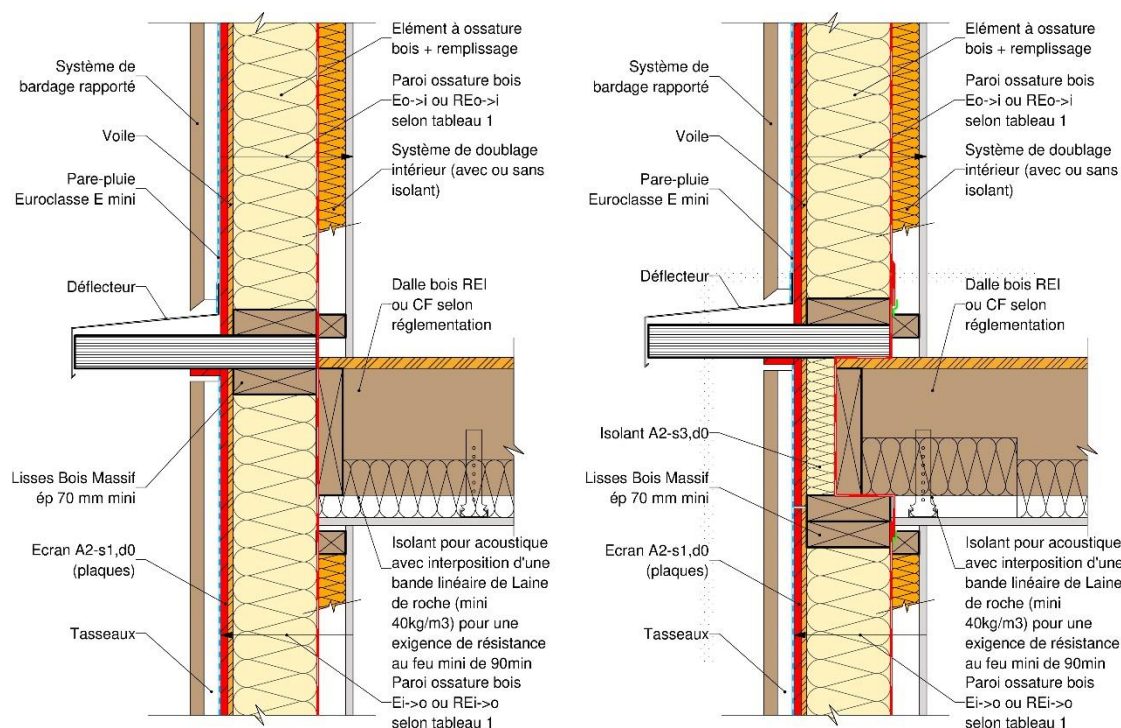
Figure 20 : Exemple de paroi avec déflecteurs renforcés d'une Façade/mur ossature bois & plancher en ossature bois.
