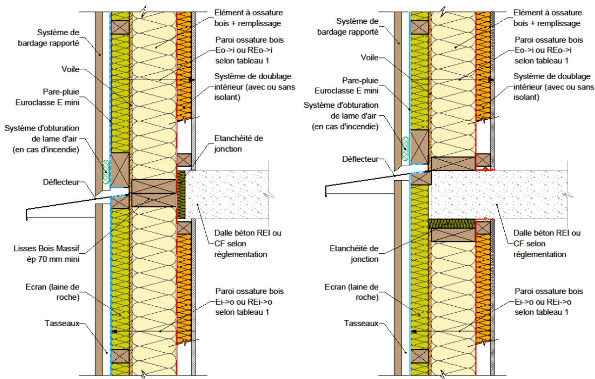
Figure 22 : Façade/mur ossature bois & plancher béton.
