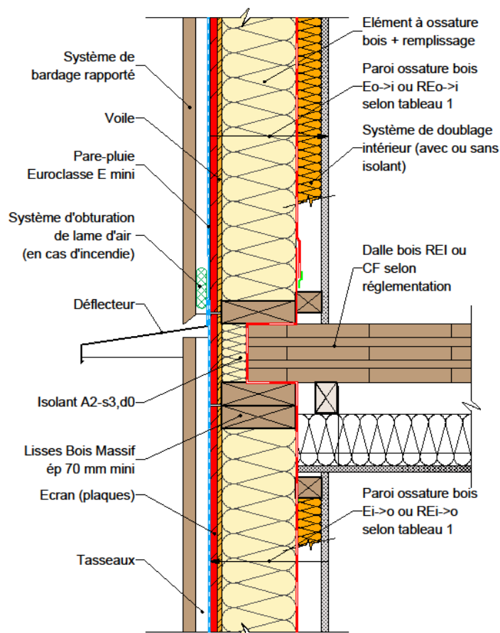
Figure 18 : Façade/mur en ossature bois & plancher en panneau bois massif.
