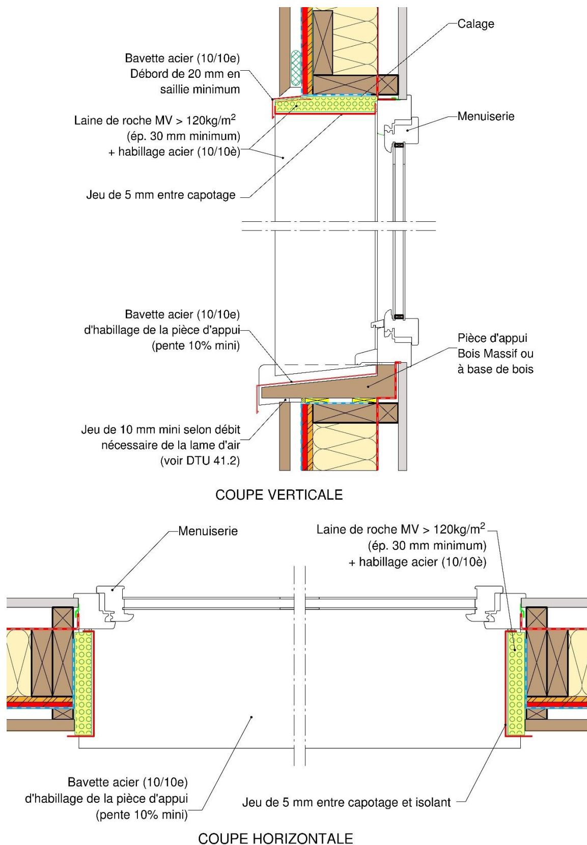
Figure 7: Traitement des embrasures de menuiseries avec un écran laine de roche + habillage acier.
