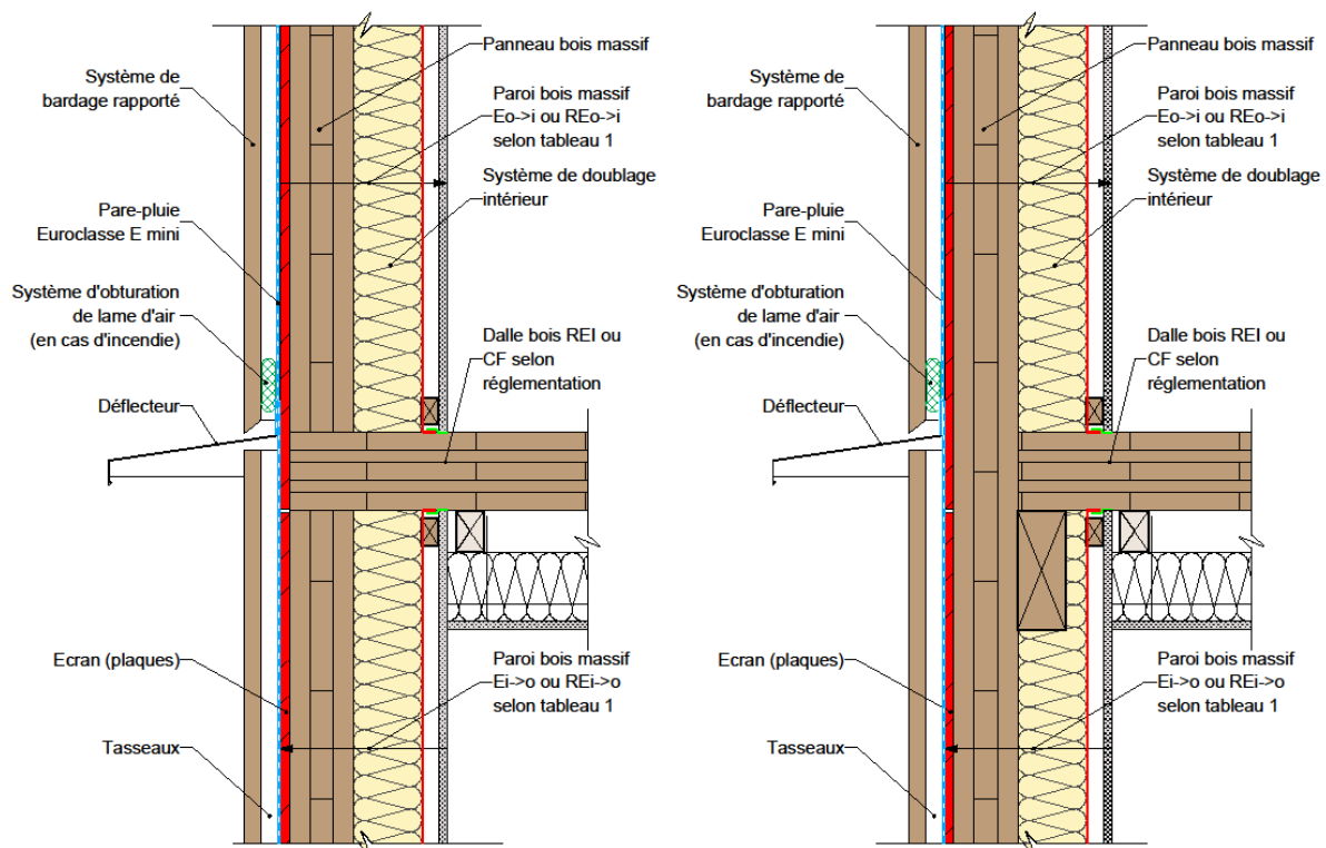
Figure 17 : Façade/mur en panneaux bois massif contrecollés et contrecloués & plancher en panneau bois massif contrecollés et contrecloués.
