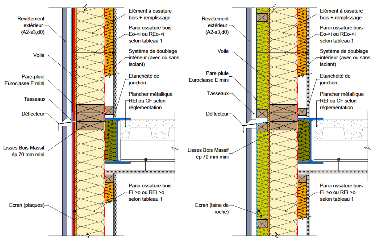
Figure 35 : Façade/mur en ossature bois & plancher métallique.
