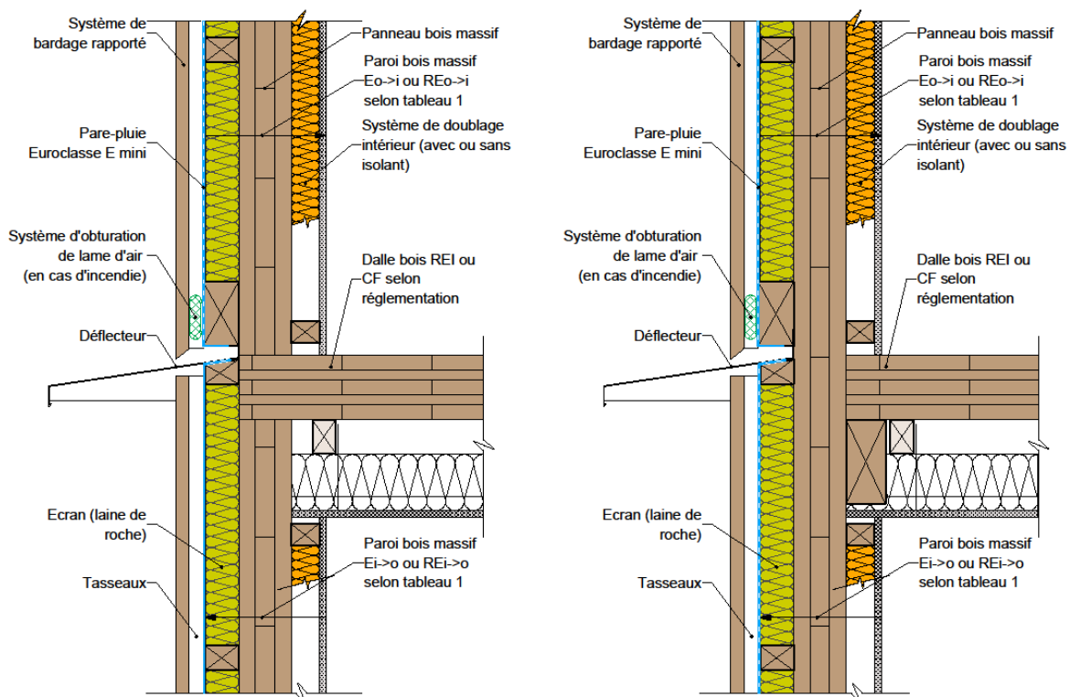
Figure 24 : Façade/mur en panneaux bois massif & plancher en panneau bois massif.
