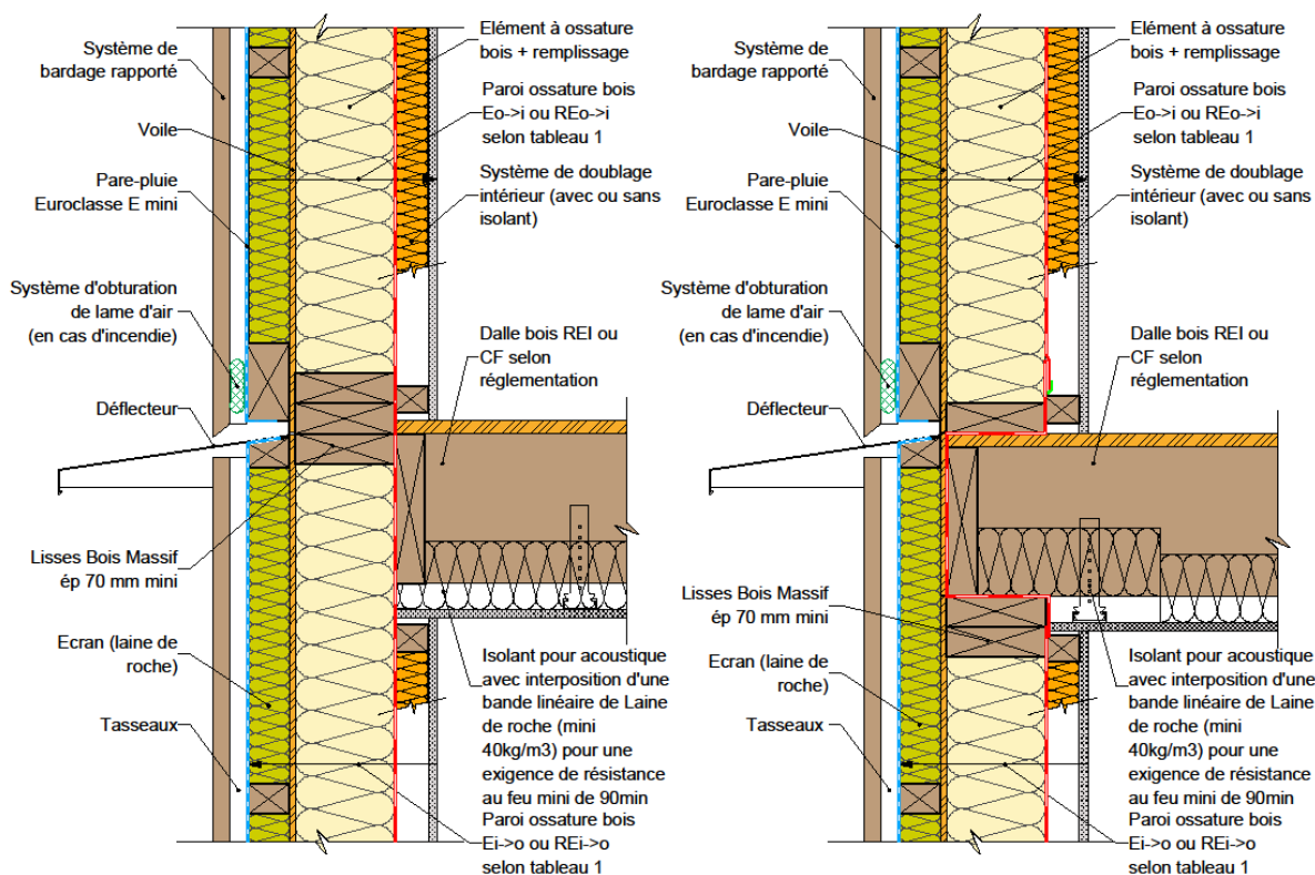
Figure 23 : Façade/mur ossature bois & plancher en ossature bois.
