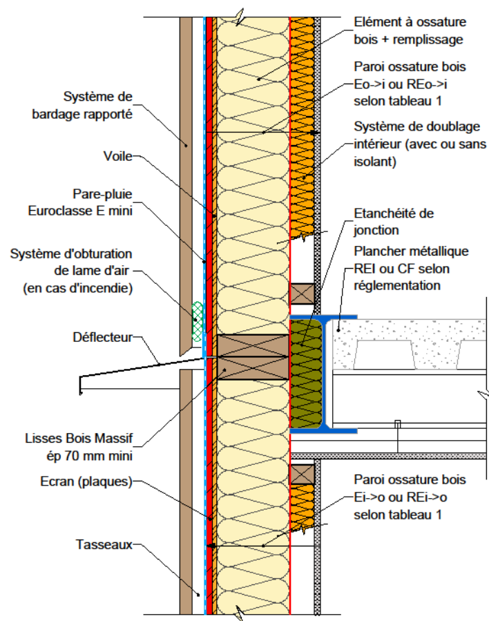
Figure 19 : Façade/mur ossature bois & plancher métallique.
