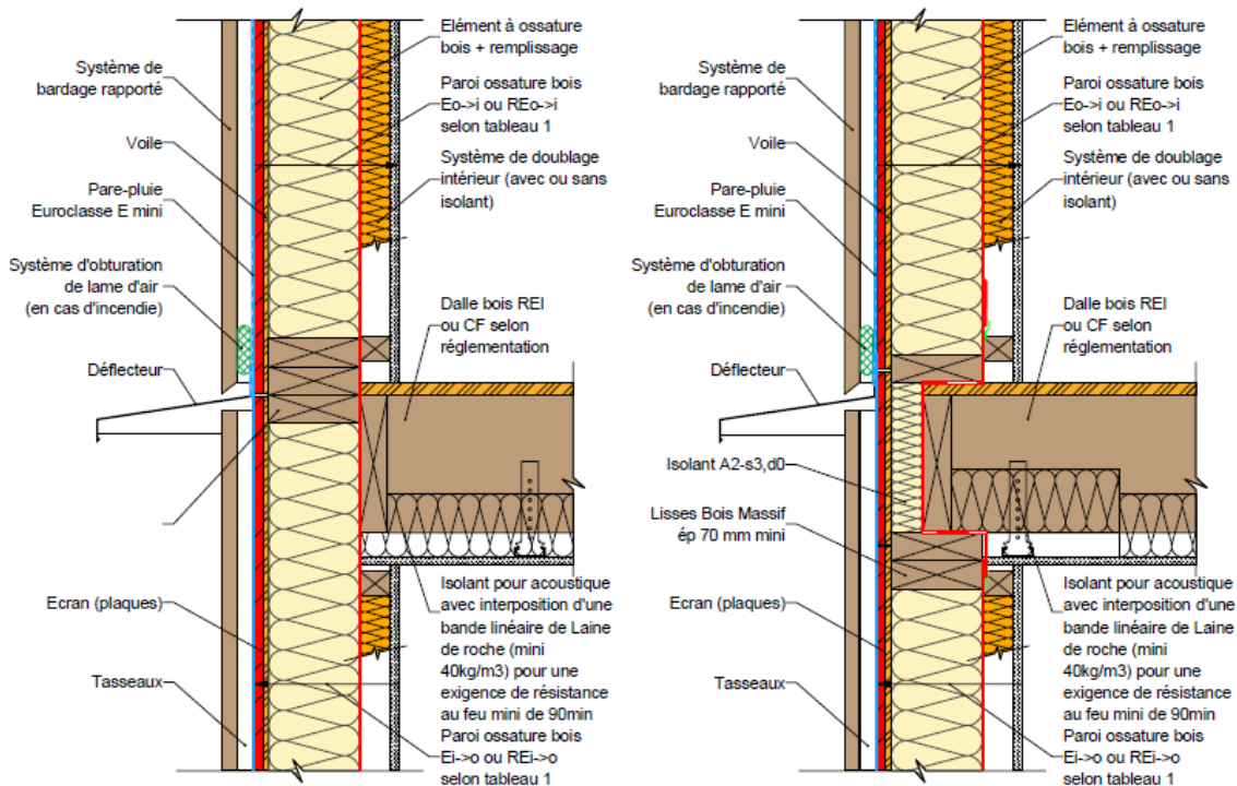
Figure 16 : Façade/mur ossature bois & plancher en ossature bois.
