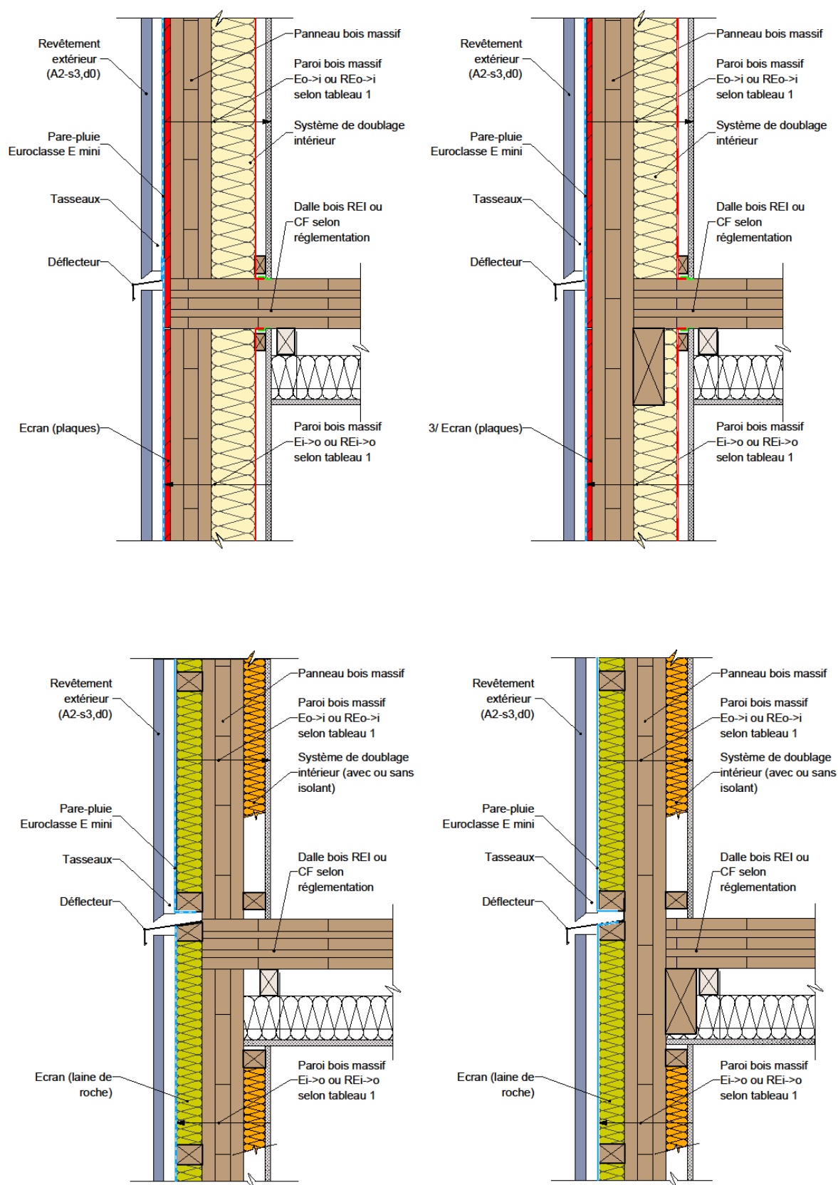
Figure 33 : Façade/mur en panneaux bois massif & plancher en panneaux bois massif.
