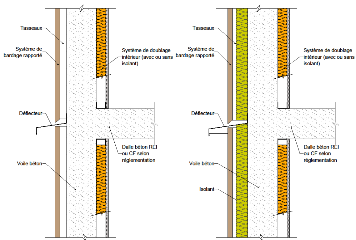
Figure 36 : Bardage ventilé avec revêtement extérieur à base de bois sur support en maçonnerie.
